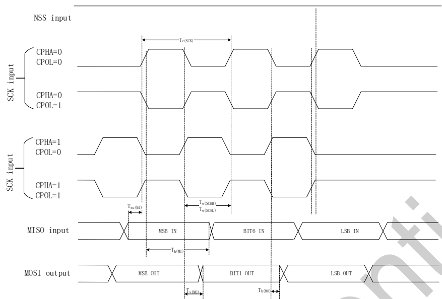
图 5-4 SPI 时序图 – 主机模式
