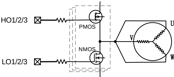
图 5-5 MOS 示意图
