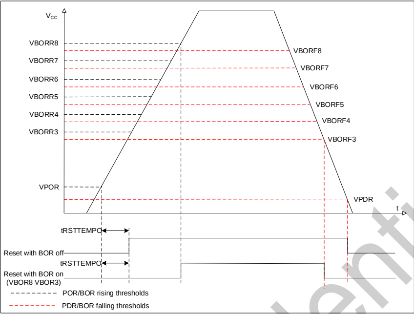
图 2-3 POR/PDR/BOR 阈值
